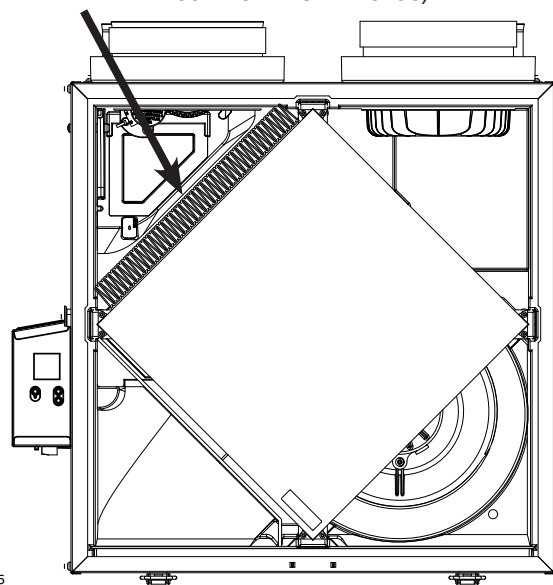
FILTRE OPTIONNEL MERV13 (FILTRE À L'ÉVACUATION NON INCLUS)
